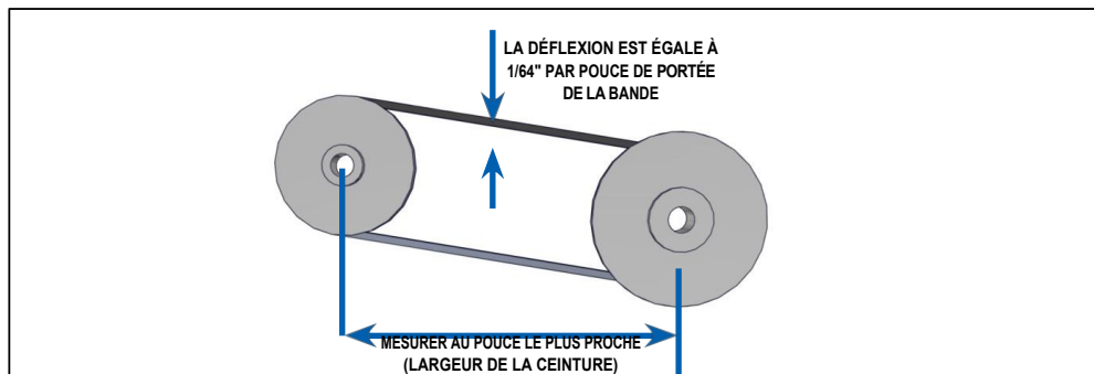
FIGURE 7.5.0 TENSION DE LA COURROIE DU VENTILATEUR
