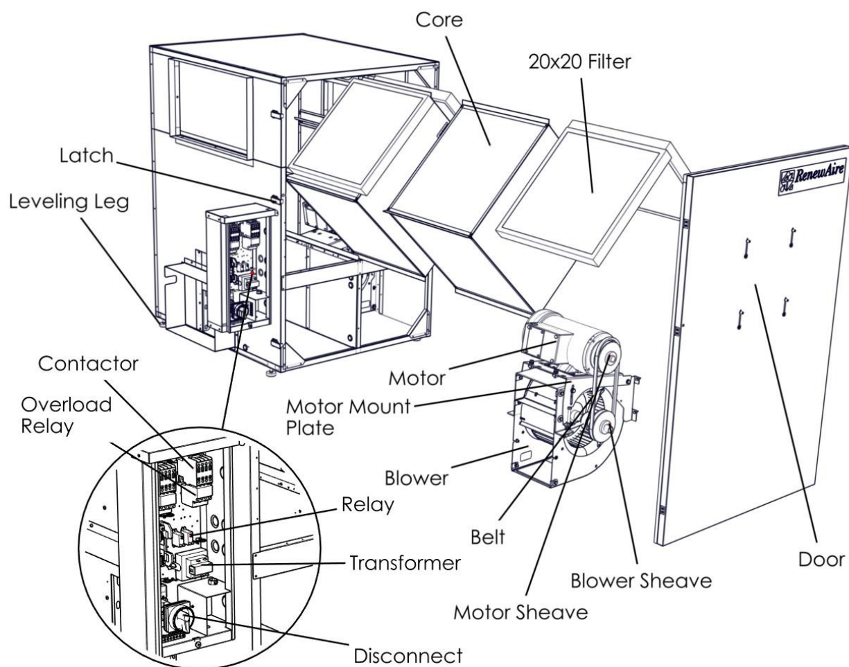
FIGURE 7.8.1 PIÈCES DE RECHANGE DU HE2XINV
