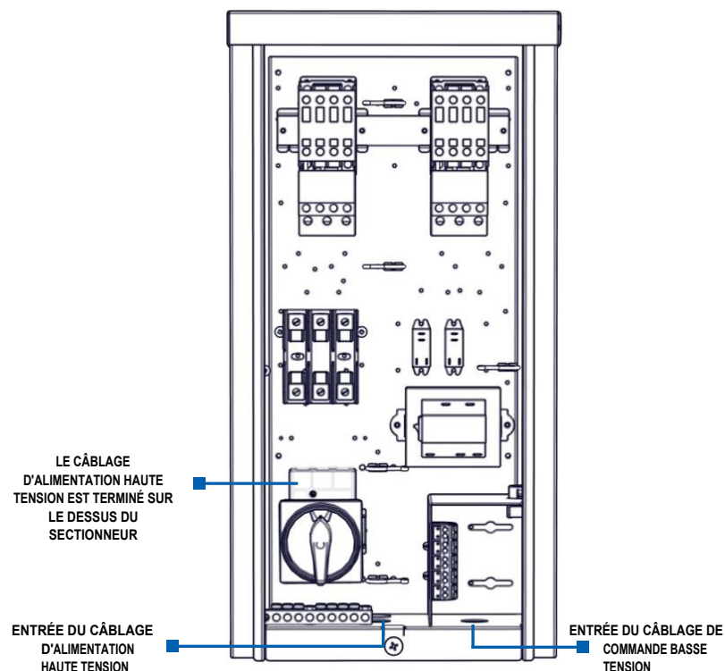
FIGURE 5.4.0 POINTS D'ENTRÉE DU CÂBLAGE DE L'E-BOX
