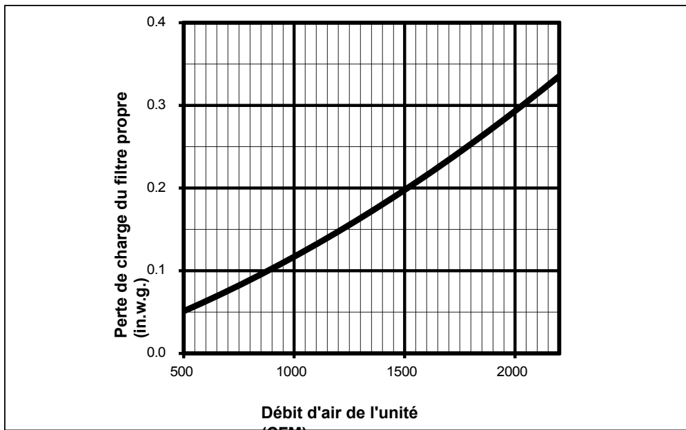
FIGURE 6.4.3 CHUTE DE PRESSION INITIALE DES FILTRES MERV 13, DISPONIBLES COMME ACCESSOIRES
