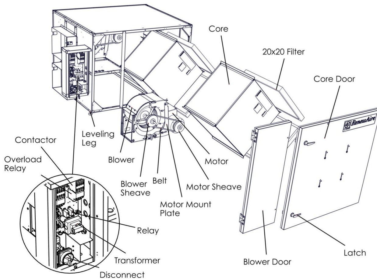
FIGURE 7.8.0 HE2XINH PIÈCES DE RECHANGE
