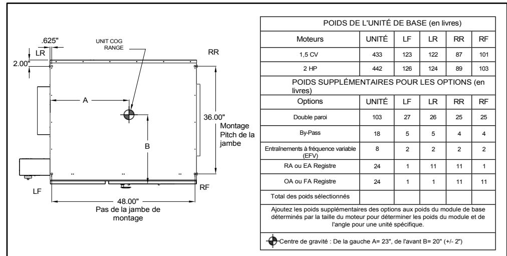
FIGURE 3.2.0 HE2XINH POIDS ET COG
