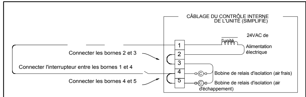
FIGURE 5.6.0 COMMANDE SIMPLE À 2 FILS, NON ALIMENTÉE
