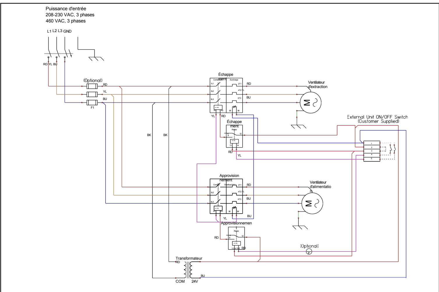
FIGURE 5.5.1 SCHEMA DE CÂBLAGE GÉNÉRIQUE TRIPHASE
