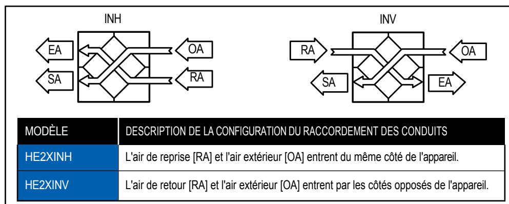
FIGURE 1.2.0 ORIENTATIONS DES FLUX D'AIR
