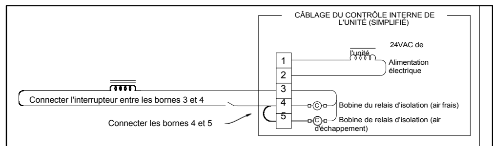
FIGURE 5.6.1 24 VAC À PARTIR D'UNE SOURCE EXTERNE
