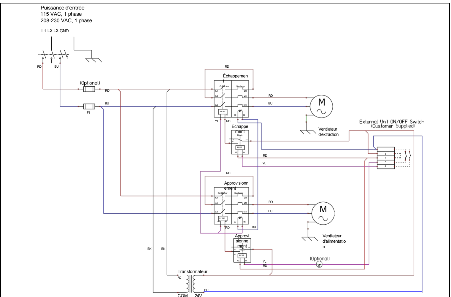
FIGURE 5.5.0 SCHEMA DE CÂBLAGE GÉNÉRIQUE MONOPHASÉ
