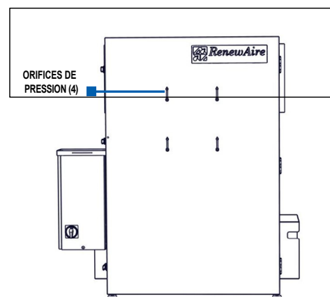
FIGURE 6.4.1 EMBLACEMENT DES PRISES DE PRESSION HE2XINV
