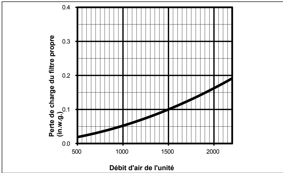
FIGURE 6.4.2 CHUTE DE PRESSION INITIALE DES FILTRES MERV 8, FOURNIS AVEC CET APPAREIL
