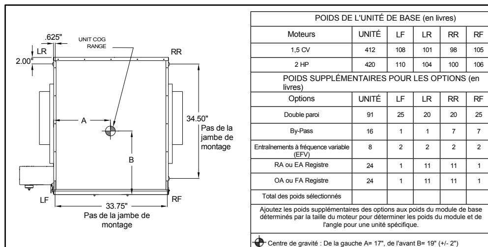
FIGURE 3.2.1 POIDS ET COG HE2XINV
