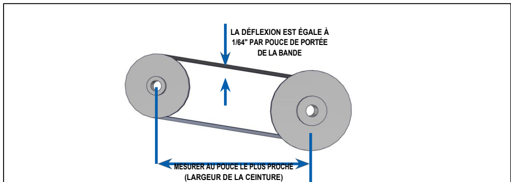
FIGURE 7.5.0 TENSION DE LA COURROIE DU VENTILATEUR
