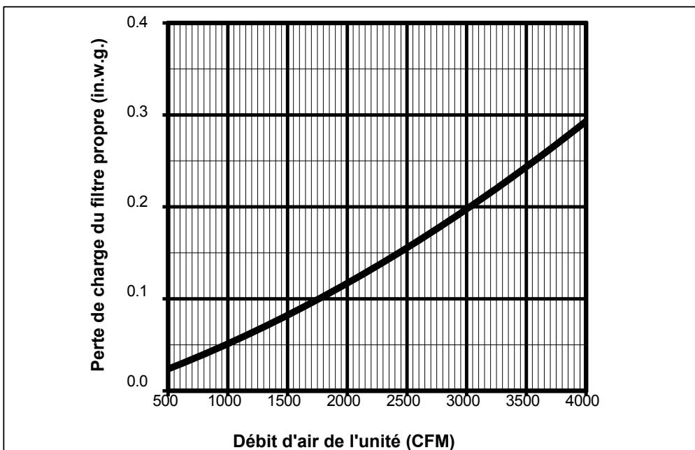
FIGURE 6.4.1 CHUTE DE PRESSION INITIALE DES FILTRES MERV 8, FOURNIS AVEC CET APPAREIL
