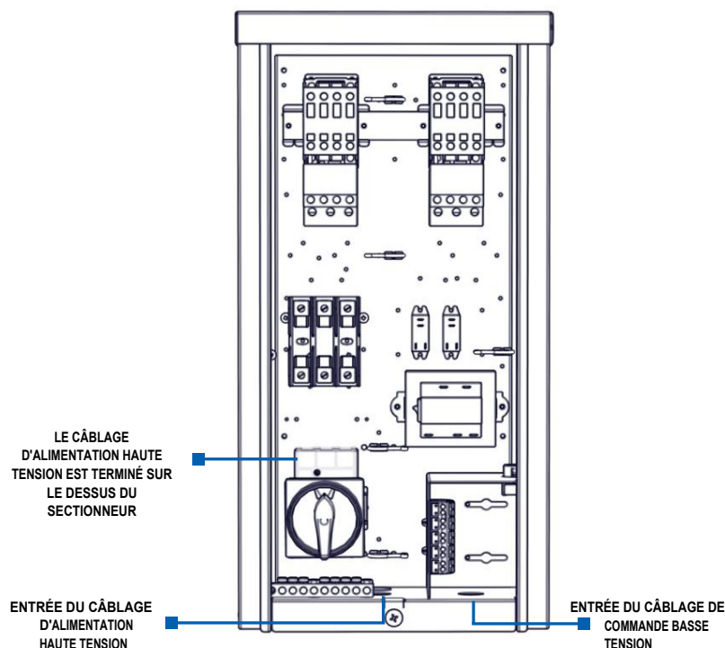
FIGURE 5.4.0 POINTS D'ENTRÉE DU CÂBLAGE DE L'E-BOX
