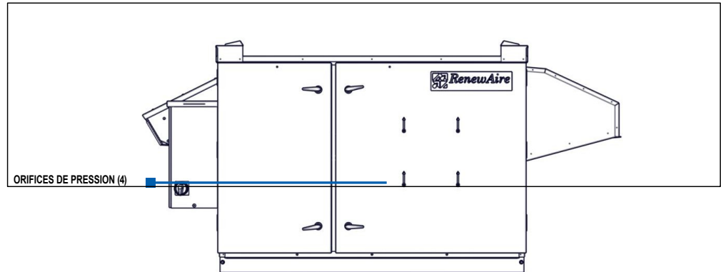
FIGURE 6.4.0 HE4XRT EMPLACEMENT DES PRISES DE PRESSION
