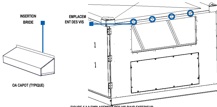
FIGURE 5.3.0 EMBLACEMENT DES VIS D'AIR EXTERIEUR
