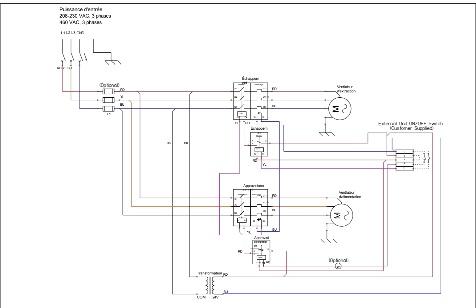
FIGURE 5.5.1 SCHÉMA DE CÂBLAGE GÉNÉRIQUE TRIPHASÉ
