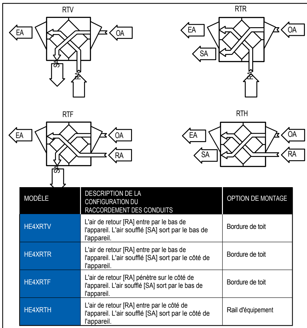
FIGURE 1.2.0 ORIENTATIONS DES FLUX D'AIR
