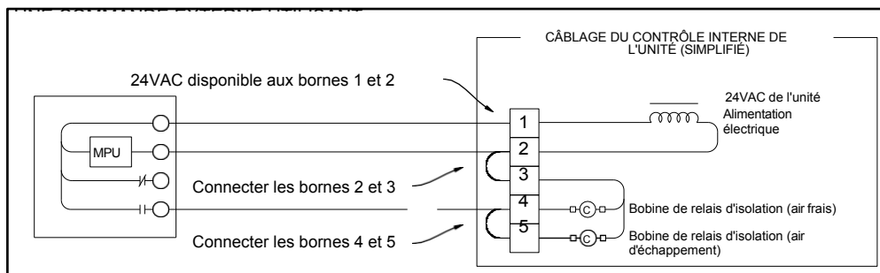
FIGURE 5.6.2 COMMANDE EXTERNE UTILISANT ERV 24 VAC
