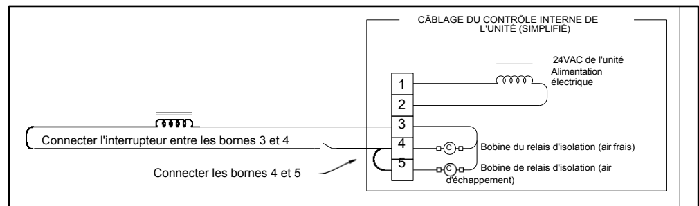
FIGURE 5.6.1 24 VAC À PARTIR D'UNE SOURCE EXTERNE
