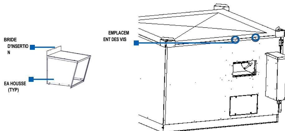
FIGURE 5.3.2 EMPLACEMENT DES VIS D'ÉVACUATION D'AIR
