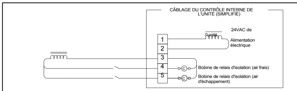
FIGURE 5.6.4 COMMANDE AVEC 2 SIGNAUX "ON", ALIMENTATION EXTERNE
