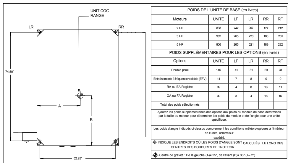
FIGURE 3.2.0 HE4XRT POIDS ET COG
