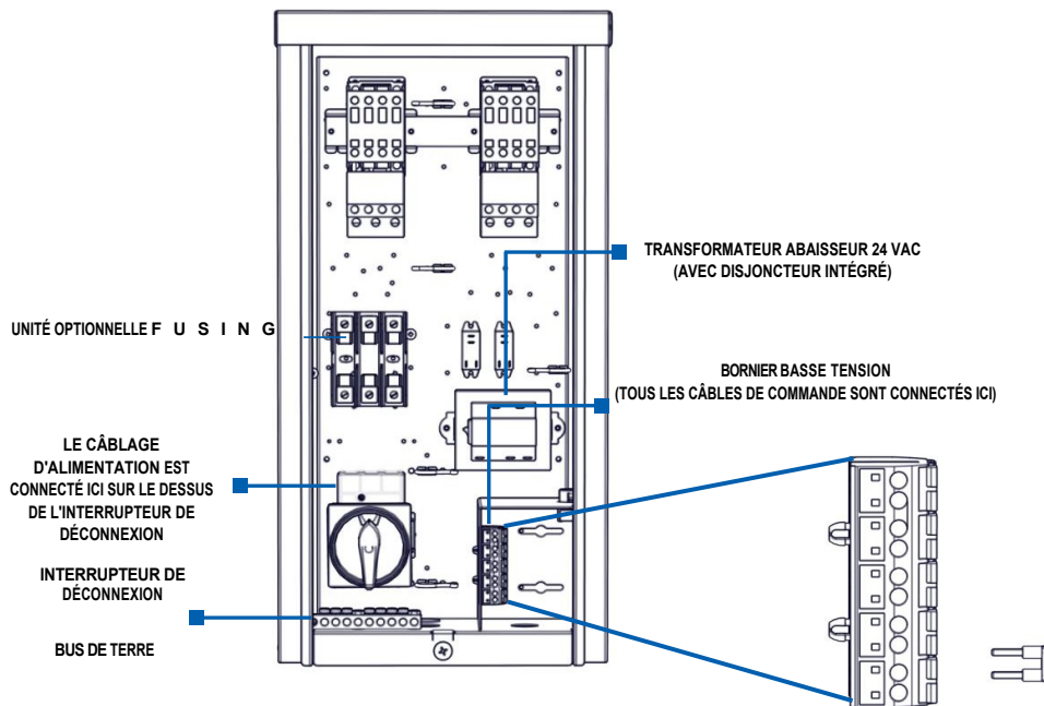
FIGURE 2.4.0 E-BOX AVEC DÉMARREURS DE MOTEURS
